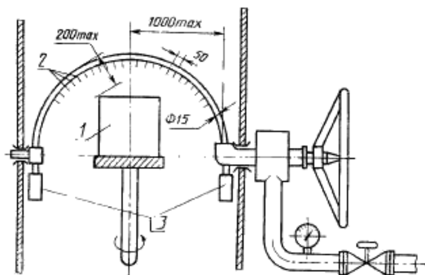
1 — испытываемая изложина; 2 — отверстия диаметром 0,4 мм; 3 — противовес
